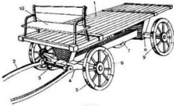
CARRO 1. Letto o pianale; 2. timone; 3. sterzo; 4. assale; 5. ruota; 6. gavello; 7. telaio; 8. scannello; 9. mozzo; 10. sedile di guida
